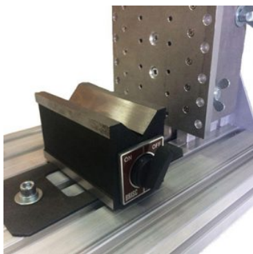
Магнитный держатель Ø30
